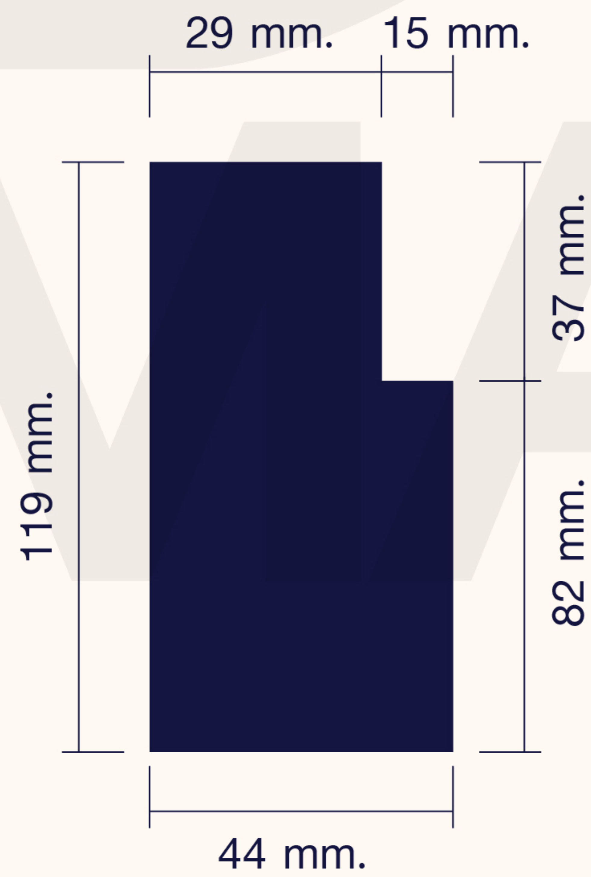
ระยะวงกบหลังไส Distance of the jamb after planing.
