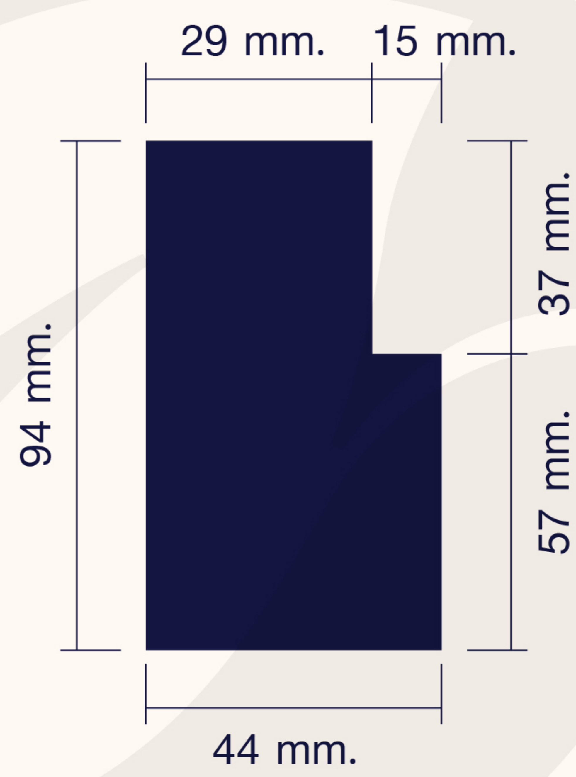
ระยะวงกบหลังไส Distance of the jamb after planing.
